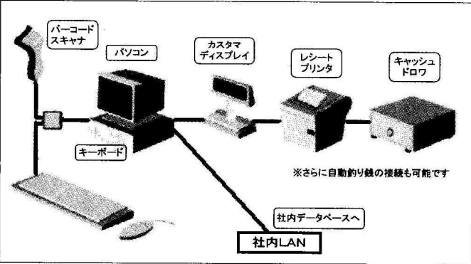
図2 PC-POSシステムの構成図
